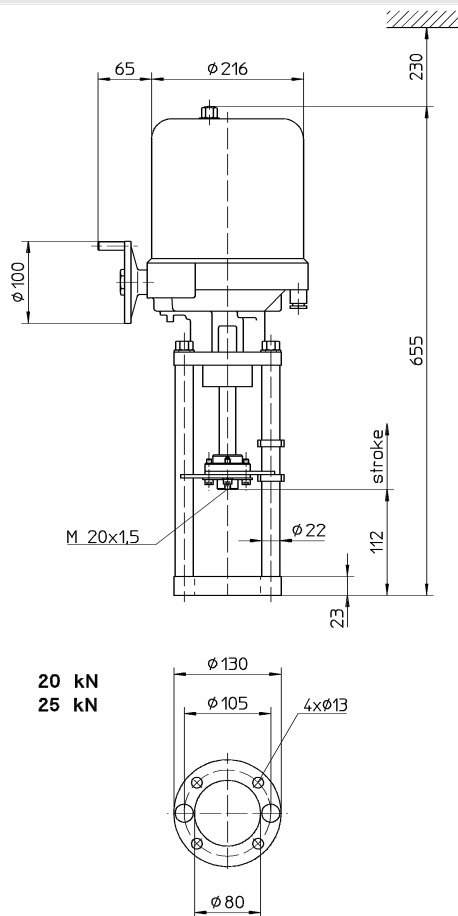
Aandrijvingen type 320.. / 325..
