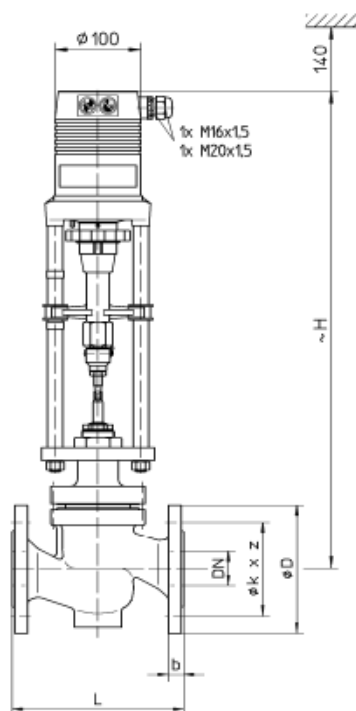
CX2F.. avec actionneurs, type 163..
