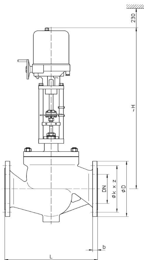
CX2F.. avec actionneur, type 320.. / 325..
