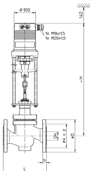
CX2F.. avec actionneurs, type 103..
